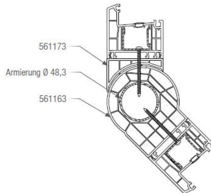
Connettore variabile
