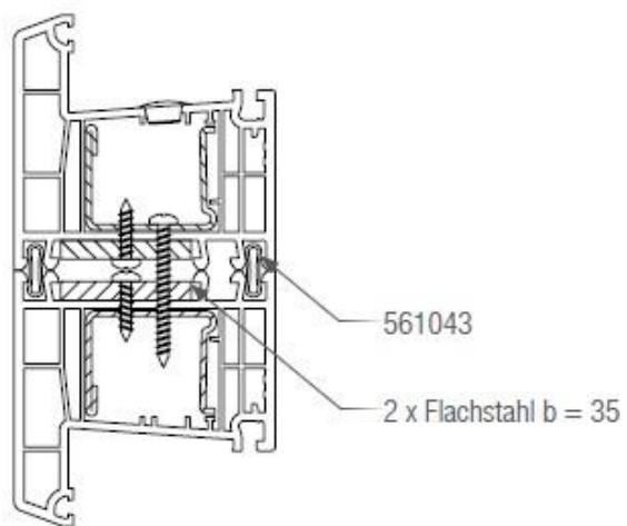
Connettore nascosto da 2 mm
