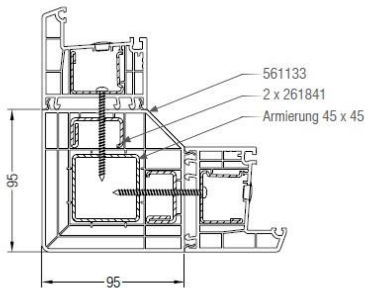
Connettore da 90 gradi
