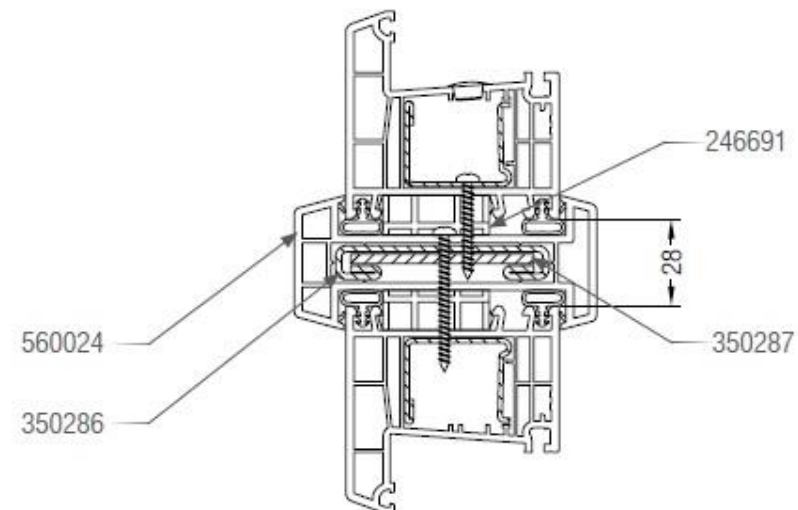
Connettore affacciato da 18 mm
